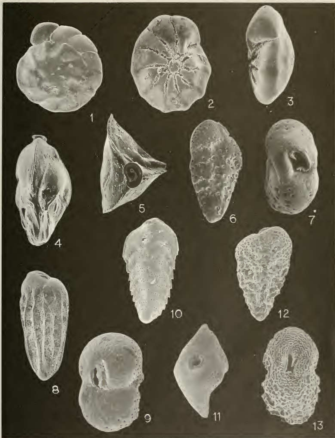
LAMINA 1. Fig. 1. Ammonia beccarii x 54, lado espiral. Fig. 2. A. beccarii x 54, lado umbilical. Fig. 3. A. beccarii x 56; vista frontal. Fig. 4. Angulogerina carinata x 77, vista lateral. Fig. 5. A. carinata x 89, vista apertural. Fig. 6. Bolivina compacta x 175, vista lateral. Fig. 7. B. compacta x 350, vista apertural. Fig. 8. Bolivina costata x 189, vista lateral. Fig. 9. B. costata x 323, vista apertural. Fig. 10. Bolivina difformis x 169, vista lateral. Fig. 11. B. difformis x 339, vista apertural. Fig. 12. Bolivina pseudoplicata x 175, vista lateral. Fig. 13. B. pseudoplicata x 269, vista apertural.
